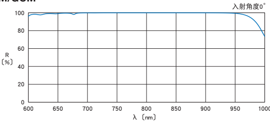
反射率波长特性 (参考数据) R: 反射率
